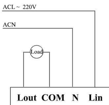
Fig. 3 BRT-803 Wiring Diagram
