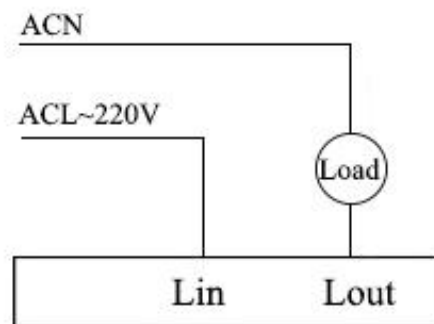
Fig. 3 BRT-800 Wiring Diagram
