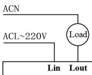
Fig. 4 BRT-403/403B wiring diagram
