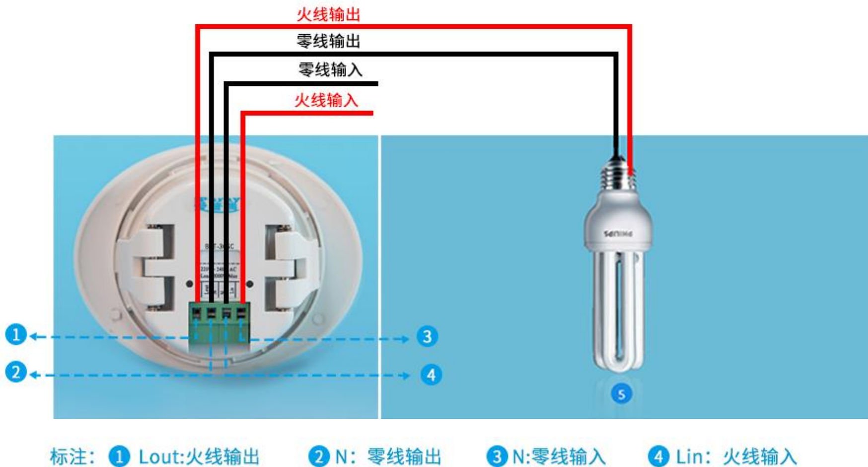
图六 BRT-306C 接线图
